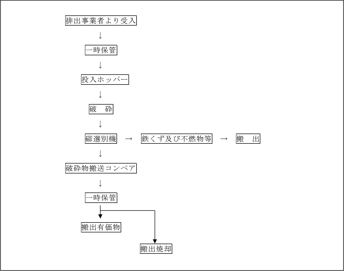
処理工程図
